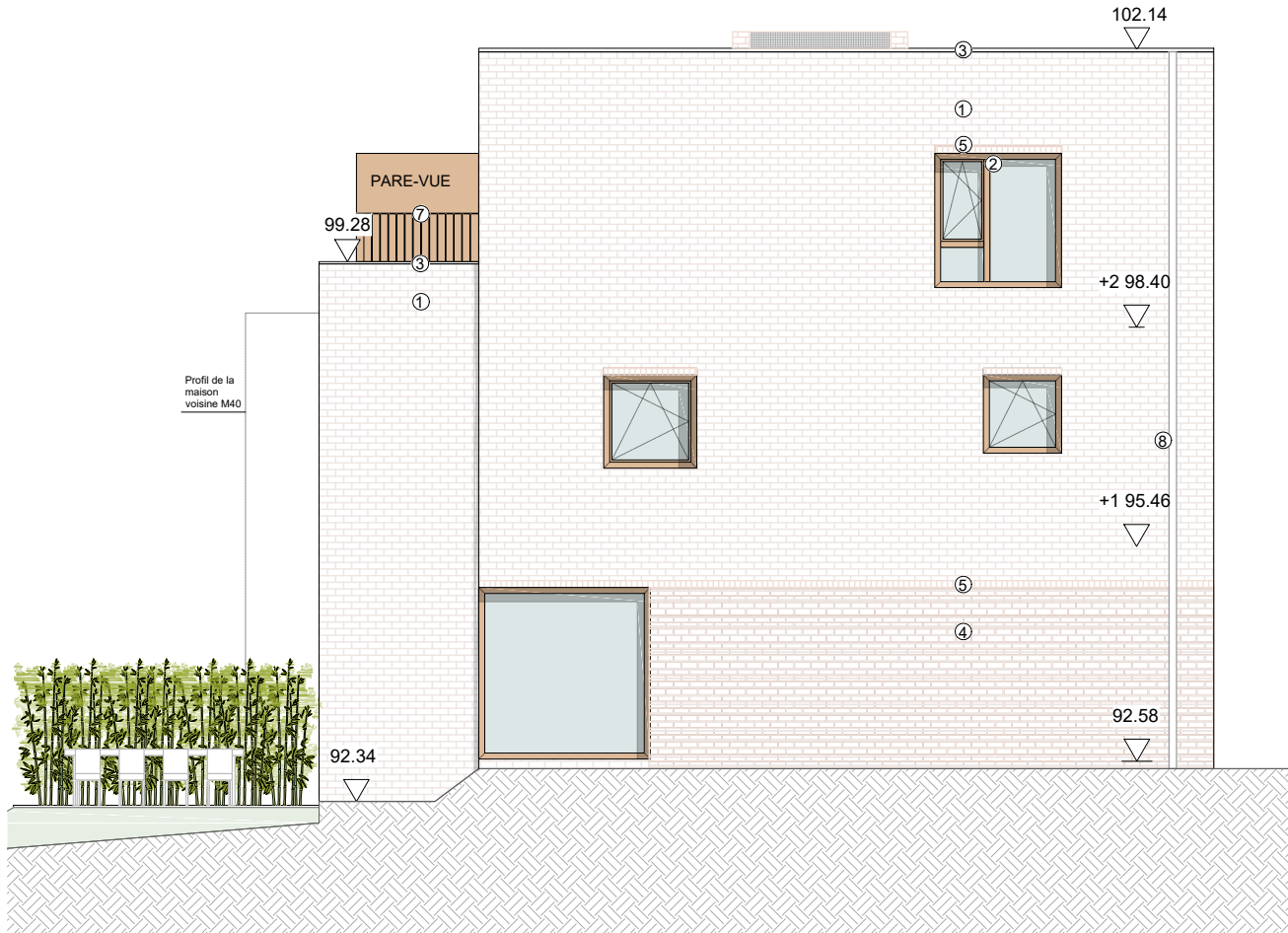
Façade sud-est / côté jardin Zuidoost gevel / tuin kant
